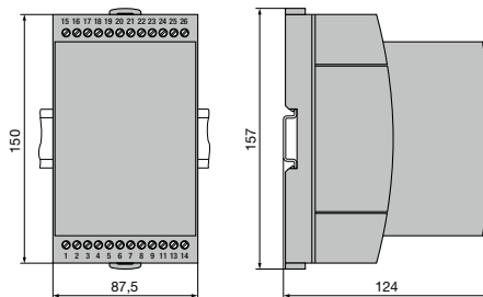
Bild 17. SINEAX DME im Gehäuse T24 auf Hutschiene (35 x 15 mm oder 35 x 7,5 mm, nach EN 50 022) aufgeschraubt.
