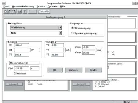
Bild 11. Programmierung der Ausgangs-Messgrößen.
