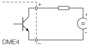
Bild 13. Prinzipschaltung für den Betrieb der Digitalausgänge.
