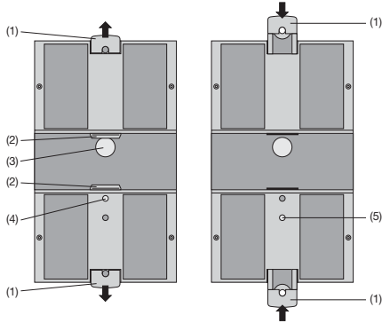
Bild 5. Geräteboden.
