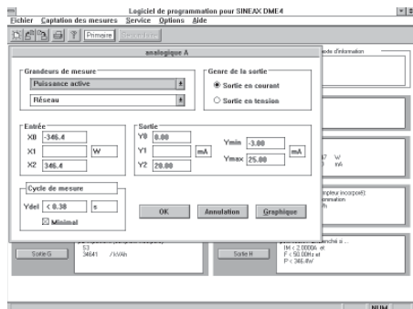
Fig. 11. Programmation des grandeurs de sortie.
