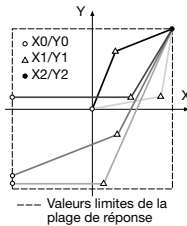
Fig. 9. Exemple des possibilités de réglage caractéristique à ligne brisée.
