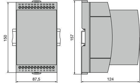
Fig. 17. SINEAX DME en boîtier T24 encliqueté sur rail «à chapeau» (35x15 mm ou 35x7,5 mm, selon EN 50 022).
