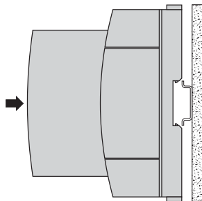
Bild 4. Montage auf Hutschiene 35 x 15 oder 35 x 7,5 mm.
