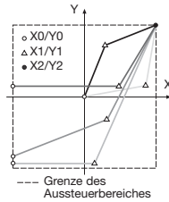
Bild 9. Beispiele für Einstellmöglichkeiten bei geknickter Kennlinie.
