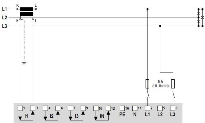
S proudovým transformátorem
