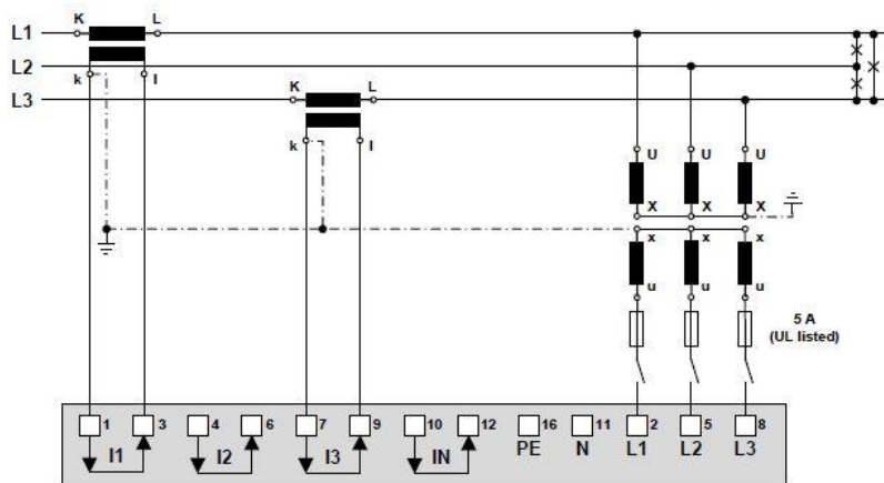
S proudovými transformátory a 3 jednopólově izolovanými transformátory napětí
