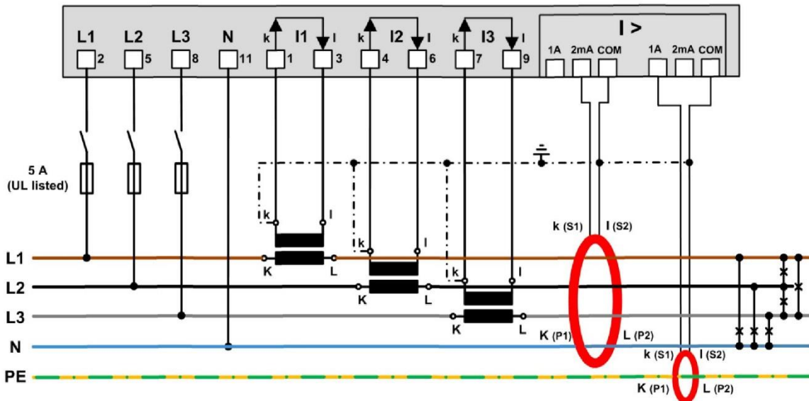
Příklad: Monitorování poruchového proudu v síti TNS
