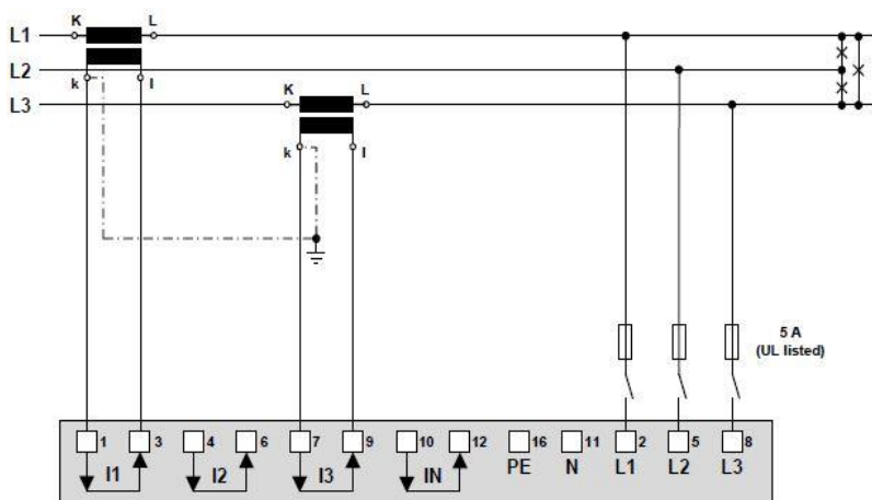
S proudovými transformátory
