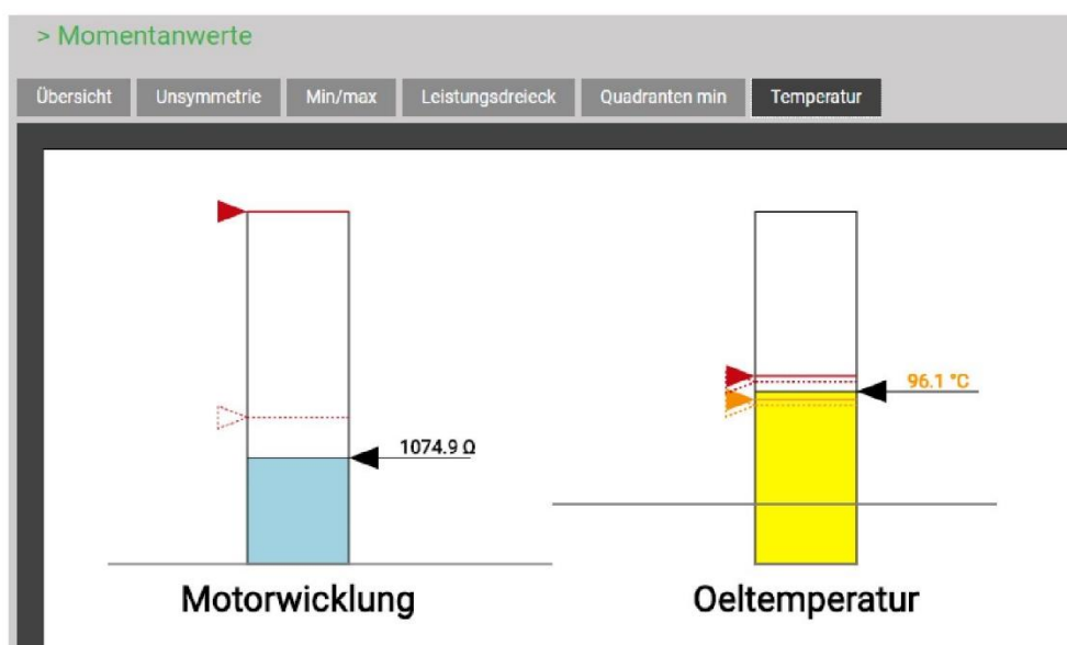
Stav monitorování teploty v menu okamžité hodnoty, PTC vlevo, Pt100 vpravo
