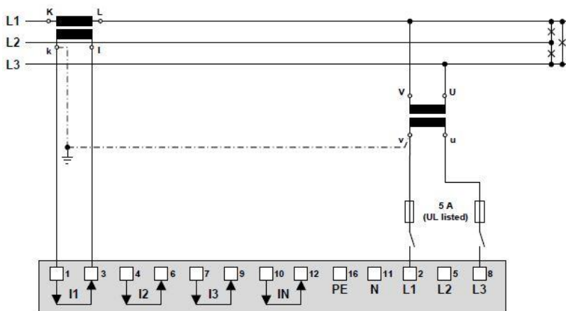
S proudovým a napěťovým transformátorem
