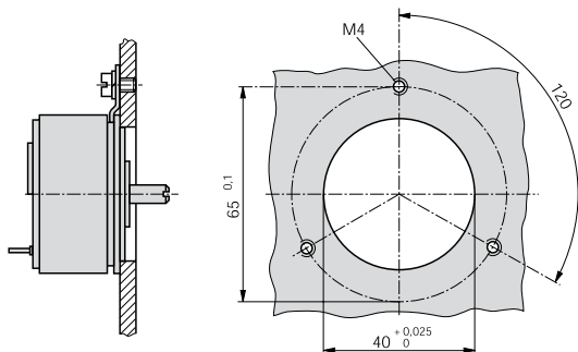
Obr. 12: Výkres vrtání pro upevnění pomocí 3 upínacích svorek
