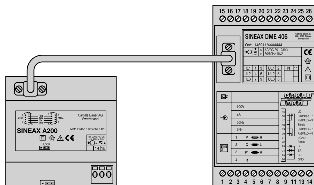
Zobrazovač A200 (pohled zezadu) spojený s DME 406 kabelem RS232.
